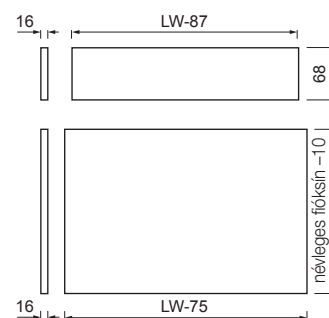
Fiókfénék és fiókhát méretezés
