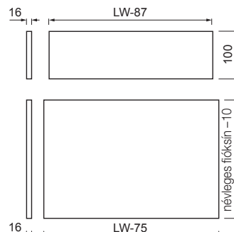
Fiókfénék és fiókhát méretezés
