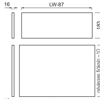
Fiókfénék és fiókhát méretezés
