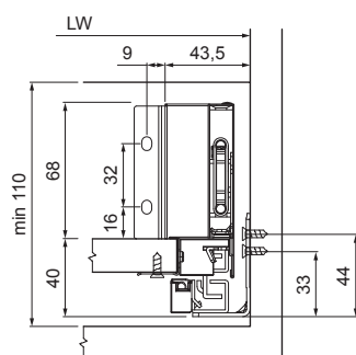
Előlaprögzítő rögzítési pontjai
