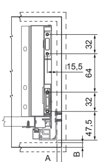
Előlaprögzítő rögzítési pontjai
